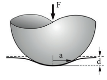
Kontakt zwischen einer Kugel und einem elastischen Halbraum
