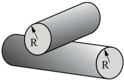
Kontakt zwischen zwei gekreuzten Zylindern mit gleichen Radien
