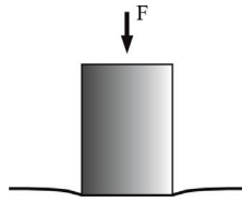
Kontakt zwischen einem starren zylindrischen Indenter und einem elastischen Halbraum
